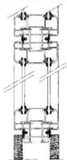
Perfil marco doble vidrio
